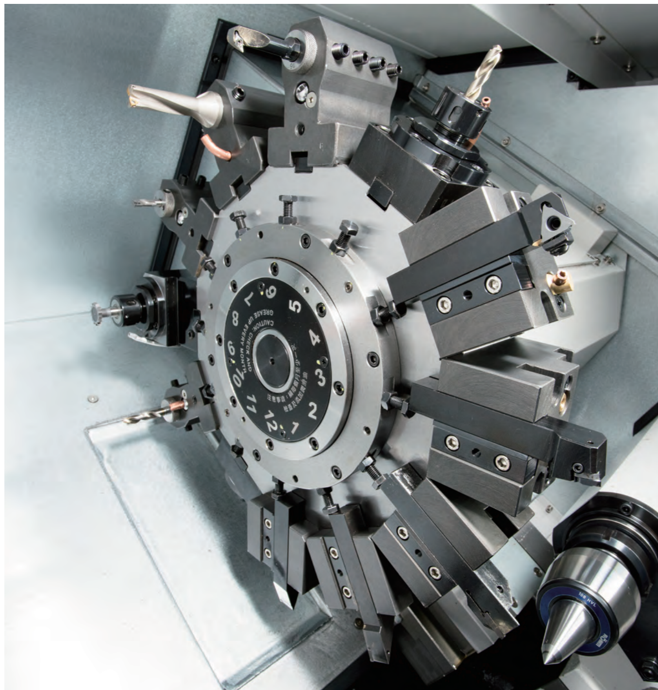
铣刀马达使用主轴马达驱动，换刀马达使用伺服马达驱动。
