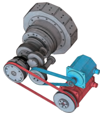
铣刀马达使用主轴马达驱动，换刀马达使用伺服马达驱动。
