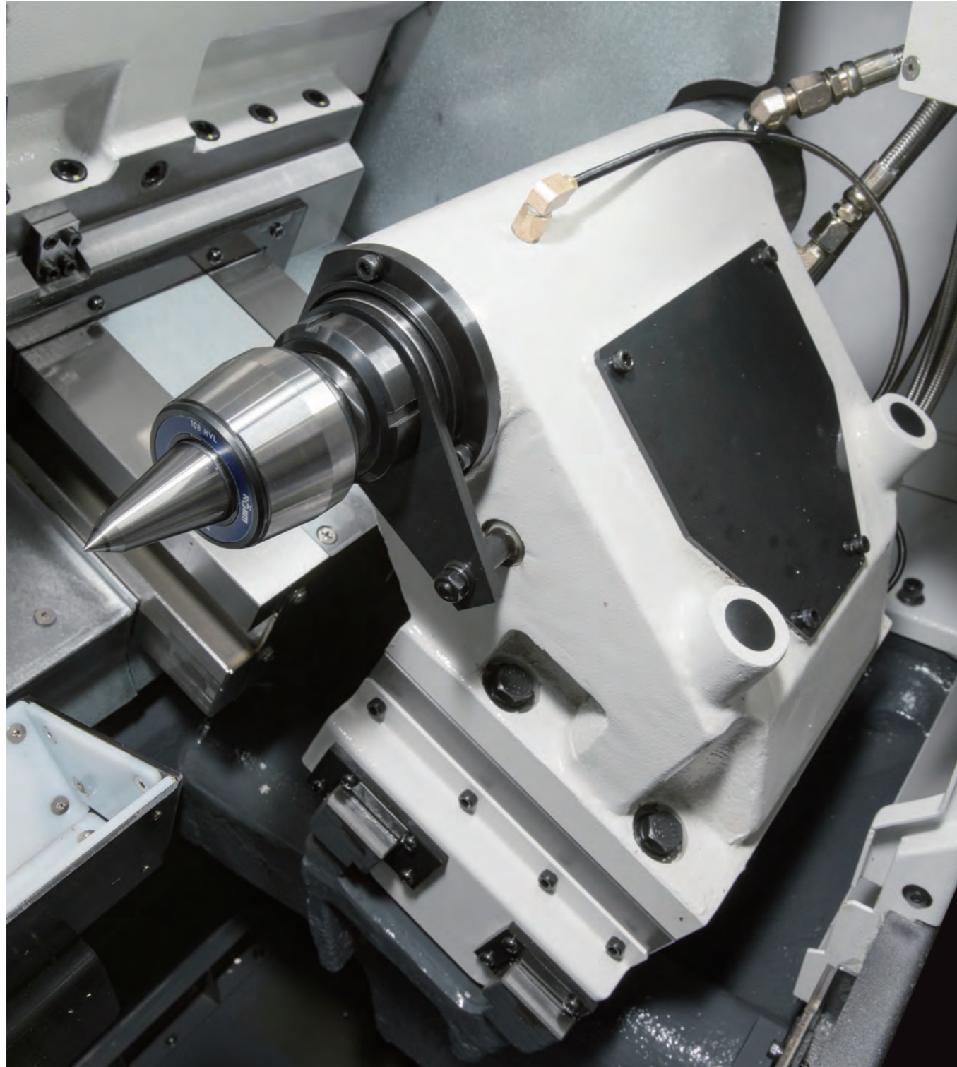
销牵引的心押台，可藉由Z轴伺服马达快速定位，缩短工时。
