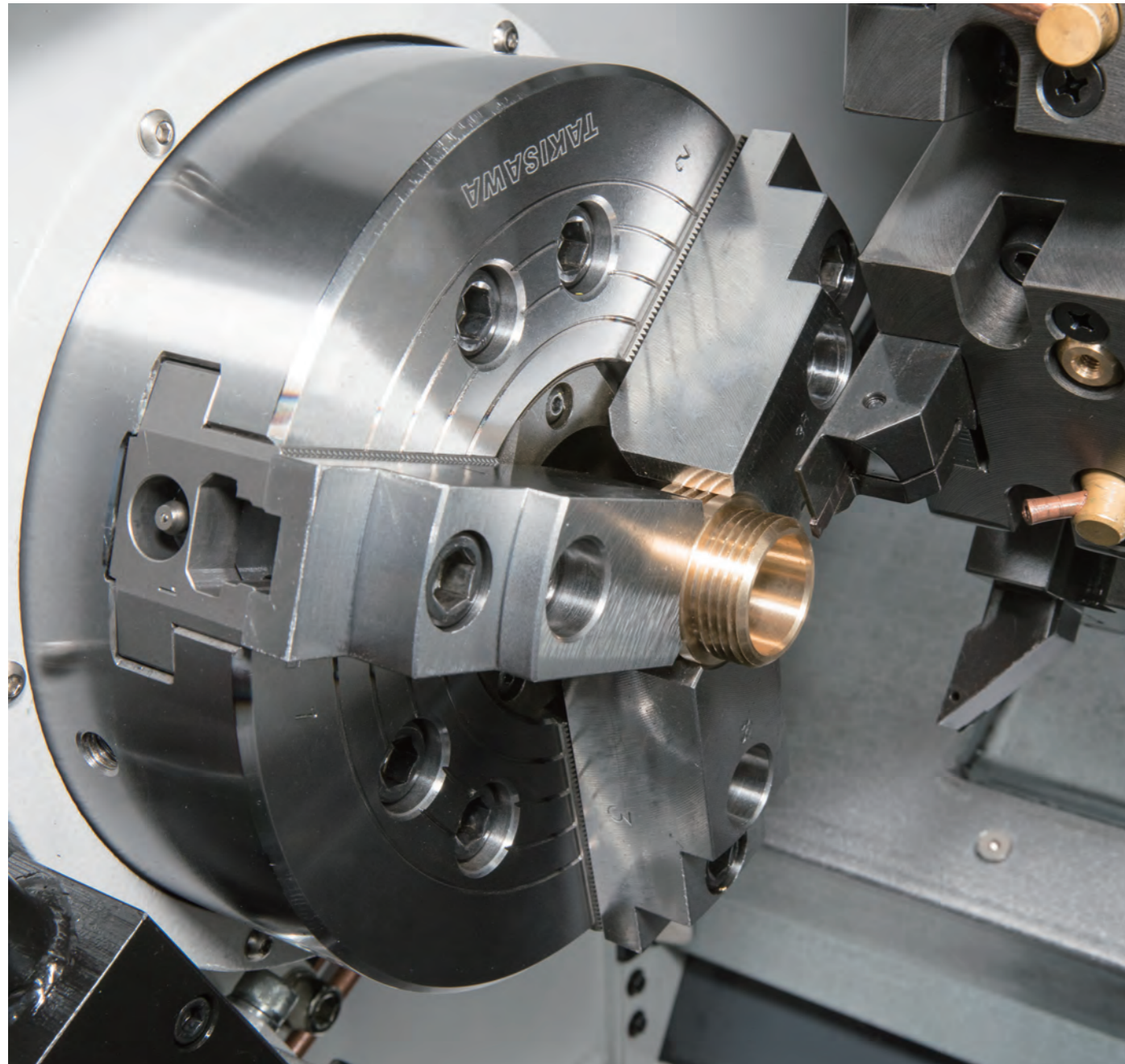
主轴使用皮带驱动，最具经济性且便于维修。
